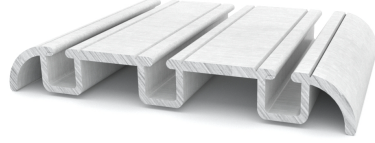
RİO BST 306 Eşikli Alt Ray Profili (3'lü) Upper Rail Profile(W/O Threshold) (0,33 kg/mt)
