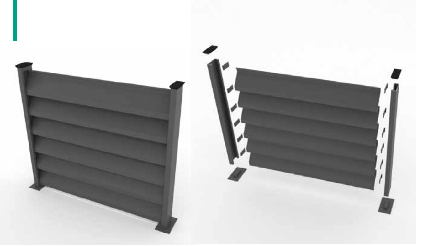
Rüzgar Kanallı Z Çit Profili / Wind Channel (Z) Type
